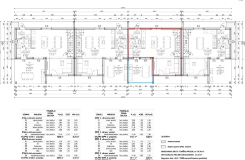
TLOČET PRIZEMLJA skala 1:100
