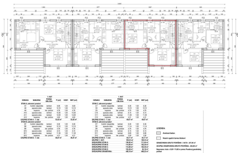
TLOČET I KATA skala 1:100
