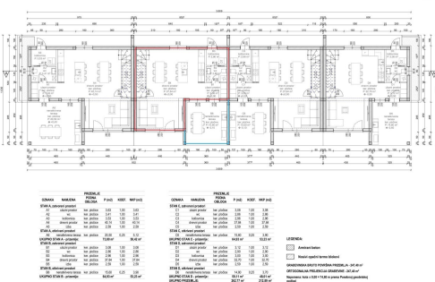
TLOCRT PRIZEMJA mjerilo 1:100
