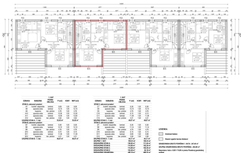
TLOCRT 1. KATA mjerilo 1:100
